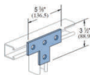
TTP-203 4 Hole Tee Plate
