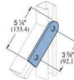
TTP-350 2 Hole Swivel Plate
