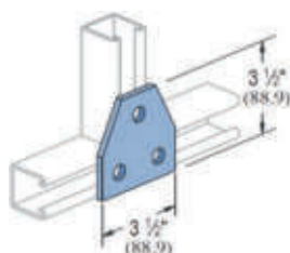
TTP-206 3 Hole Tee Corner Gusset
