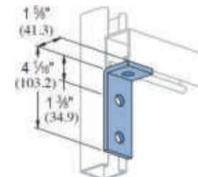
TTP-306 4 Hole Corner Angle
