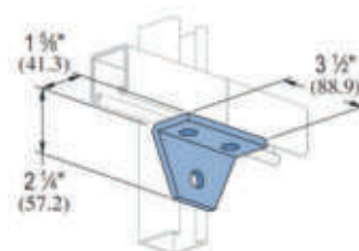
TTP-343 3 Hole Corner Joint Connector
