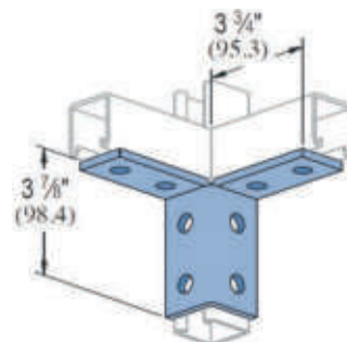
TTP-506 8 Hole Double Corner Connector
