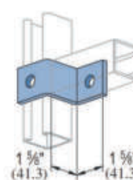
TTP-419 Offset Zee Support
