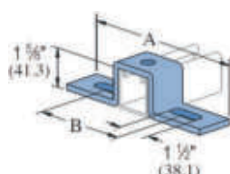
TTP-427 U Support
