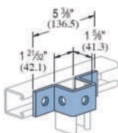
TTP-423 U Support
