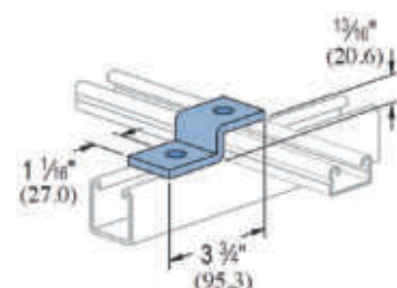
TTP-419 Offset Zee Support
