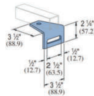
TTP-405 Slotted Corner Connector
