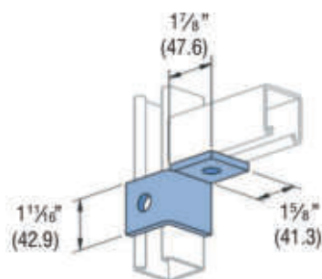
TTP-501 2 Hole Corner Connector
