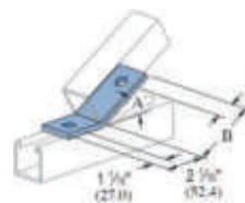
TTP-403 4 Hole Open Angle Connector
