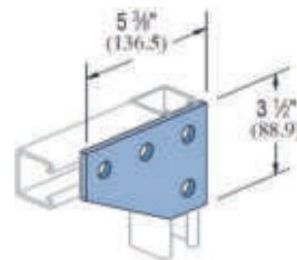
TTP-207 4 Hole Corner Gusset
