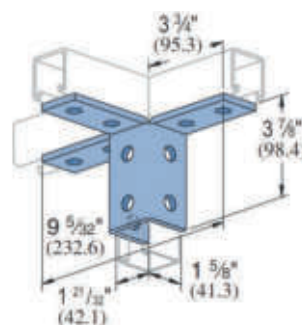
TTP-512 12 Hole Triple Connector
