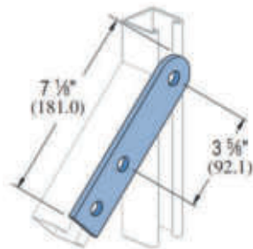
TTP-402 2 Hole Closed Angle Connector
