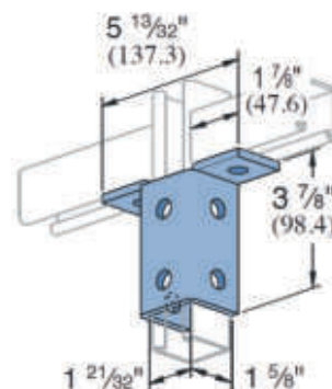
TTP-510 6 Hole Triple Wing Connector
