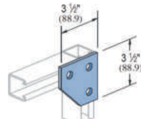
TTP-205 3 Hole Corner Gusset
