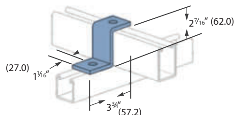
TTP-415 Zee Support
