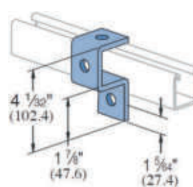
TTP-430 Cup Support for Single Strut
